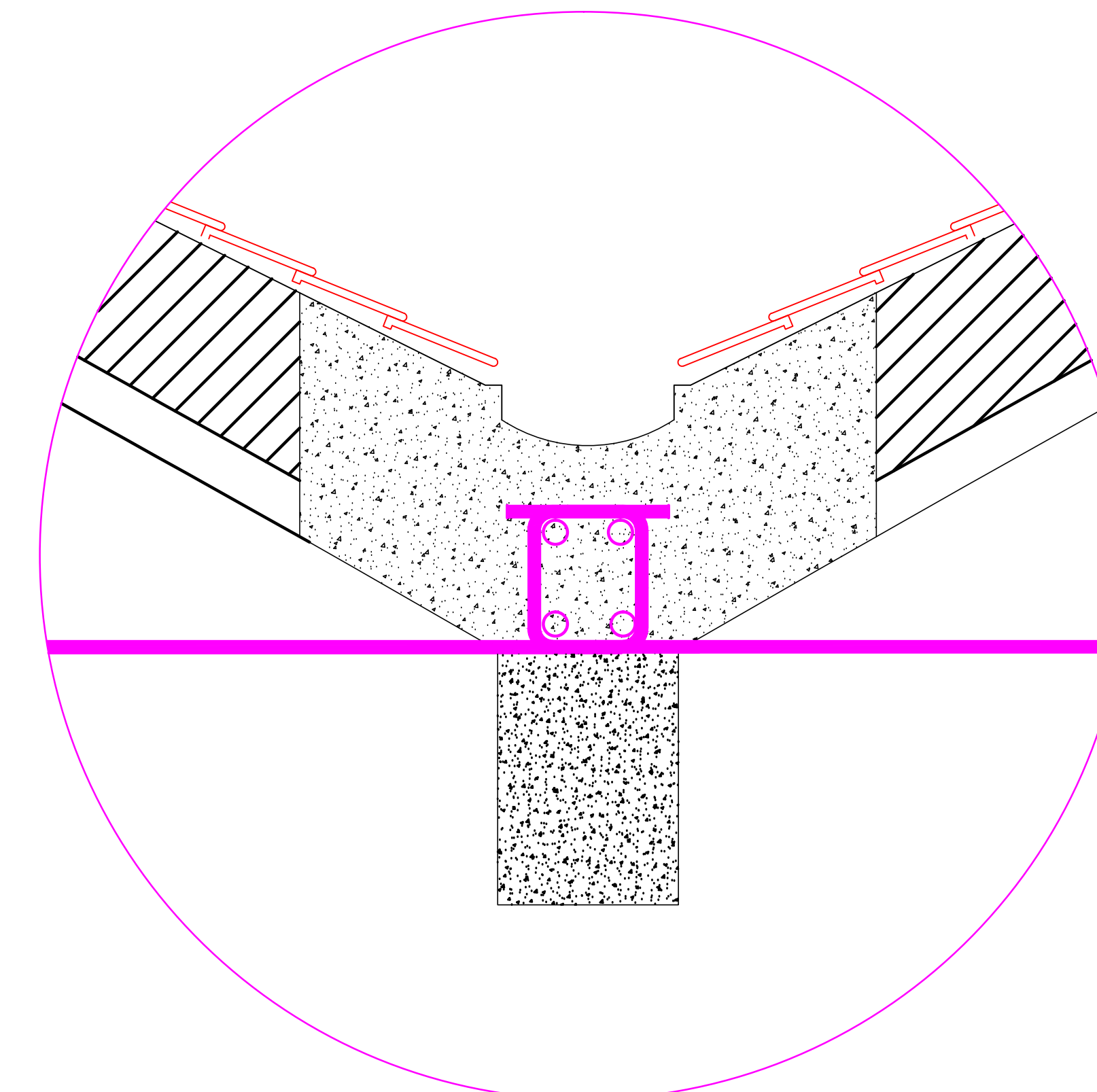
PARTICOLARE P2 - GRONDA INTERNA
