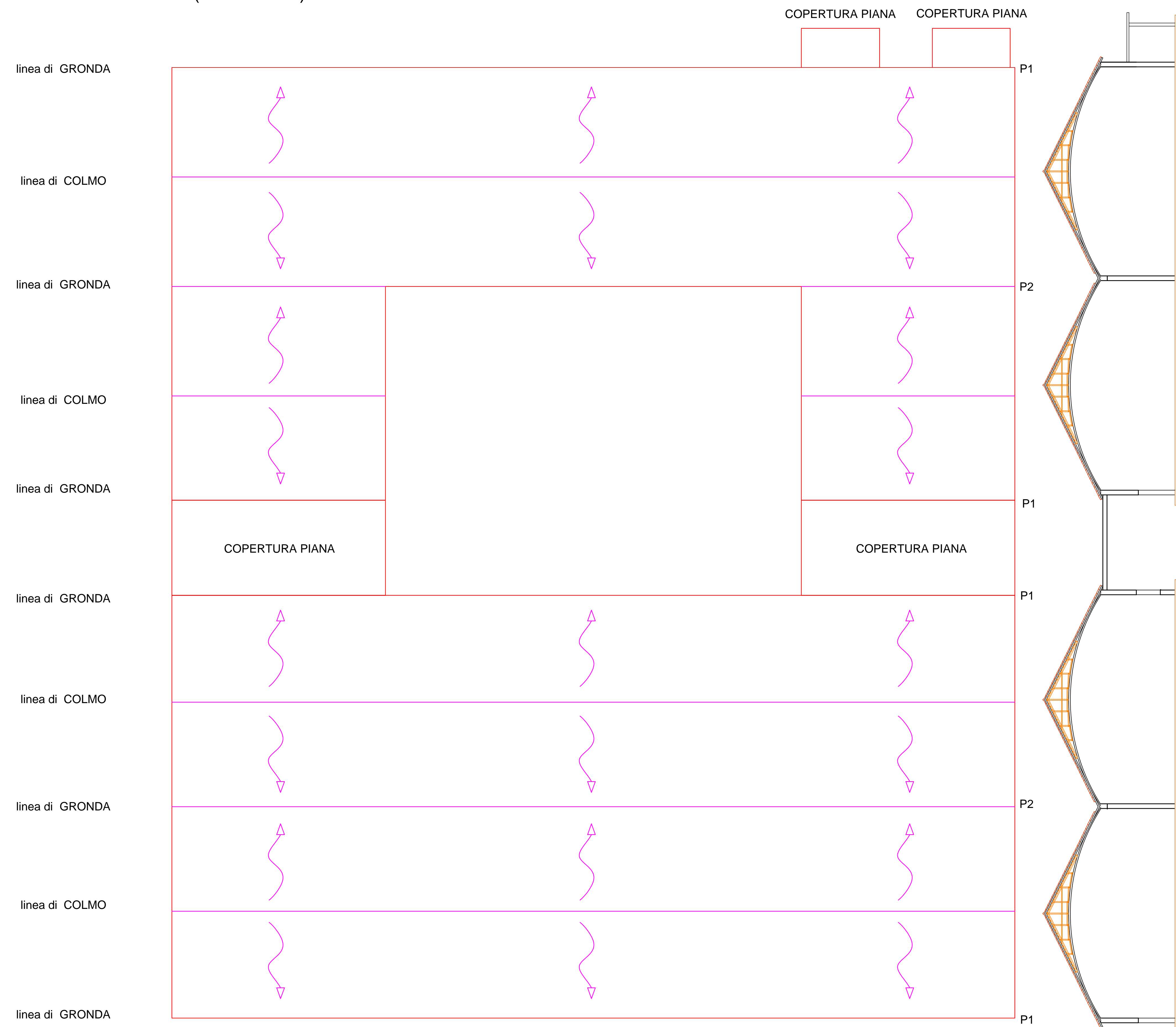
PIANTA COPERTURA (scala 1:200)
