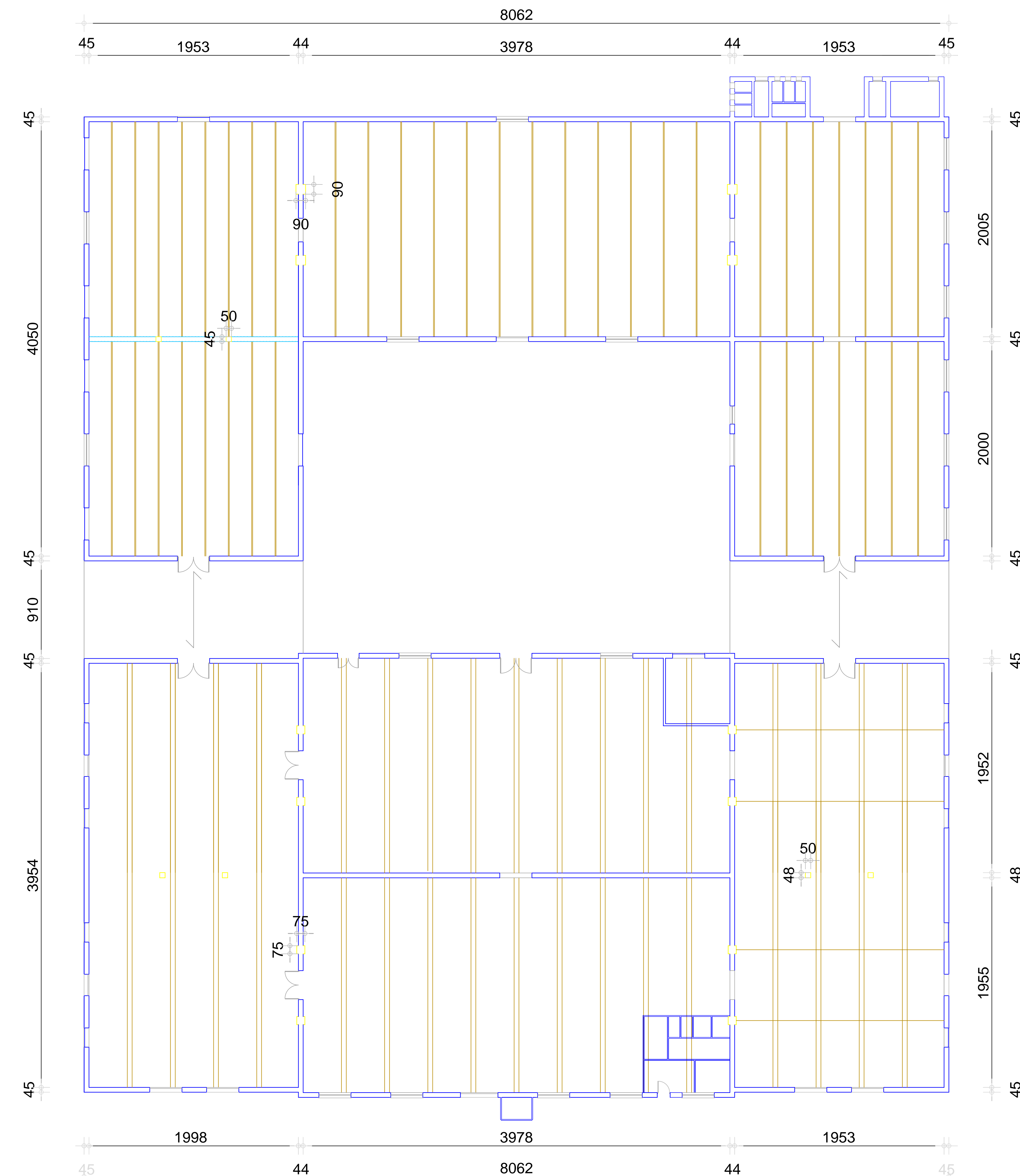
PIANTA DISPOSIZIONE TIRANTI (scala 1:200)
