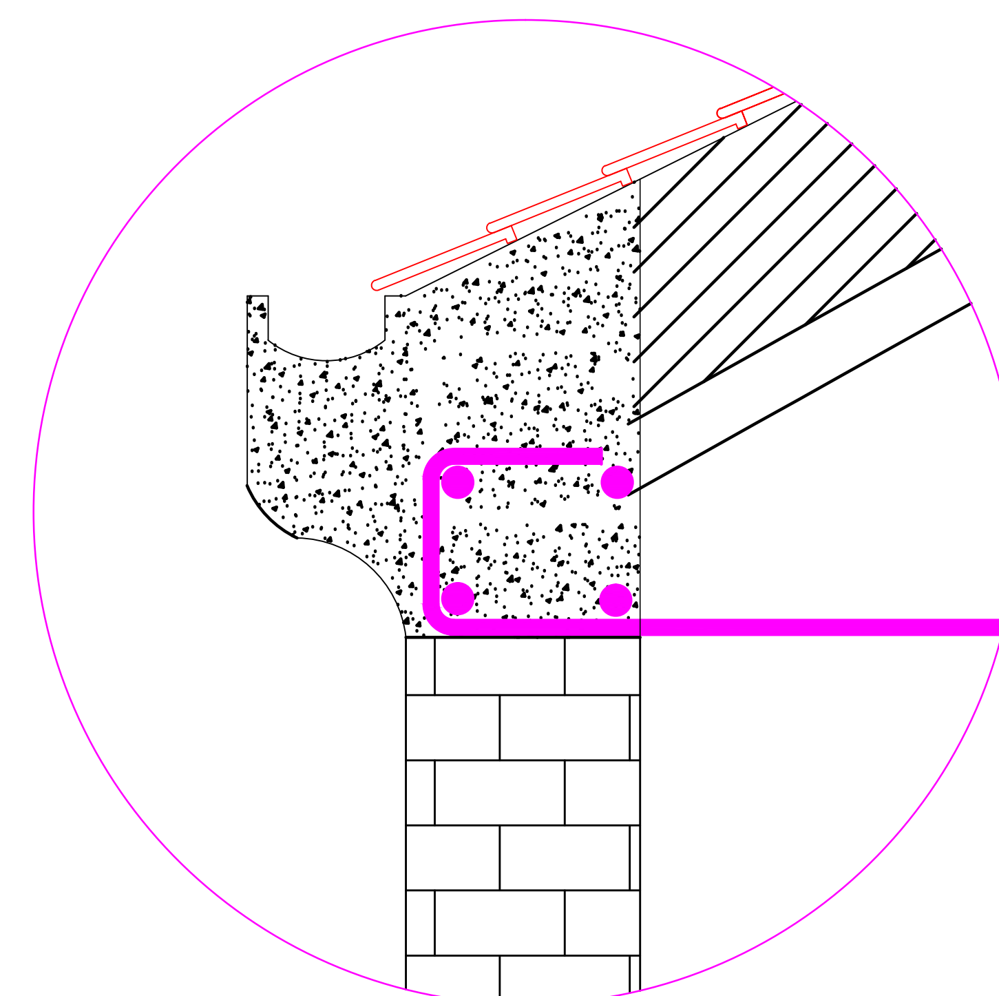
PARTICOLARE P1 - GRONDA ESTERNA
